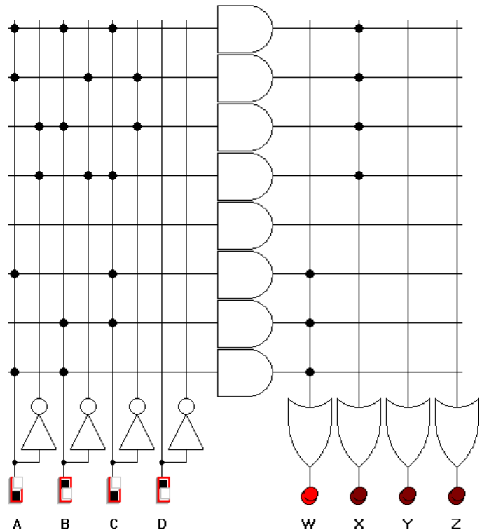
Figura 20. Sumador completo en PLA. W es el bit acarreo y X es el bit de suma.
