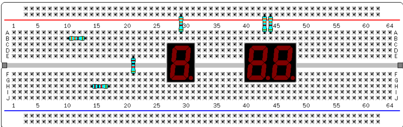
Figura 12. Resistencias y visualizadores sin funcionalidad electrónica.
