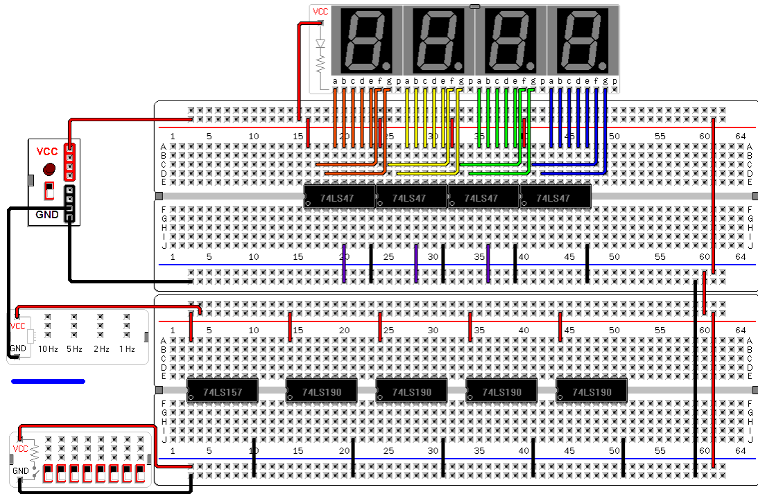
Figura 15. Conexiones de VCC y GND y de las salidas de los descodificadores a los visualizadores de siete segmentos de un contador BCD de 4 dígitos con sentido de cuenta y frecuencia seleccionables.
