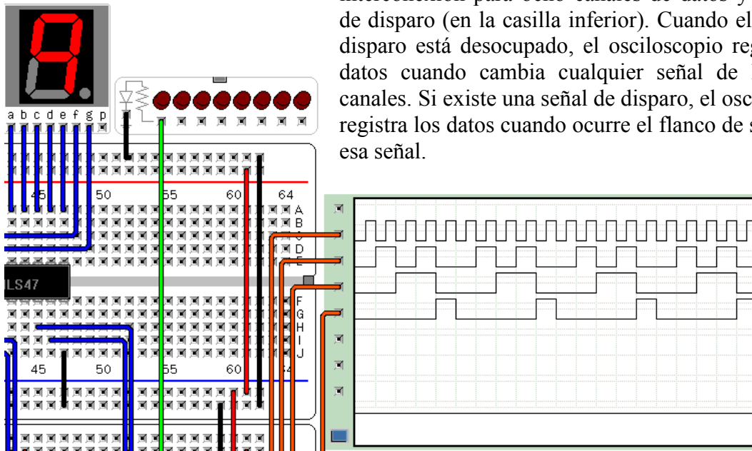
Figura 19. Visualizador en un osciloscopio del contador de unidades BCD.
